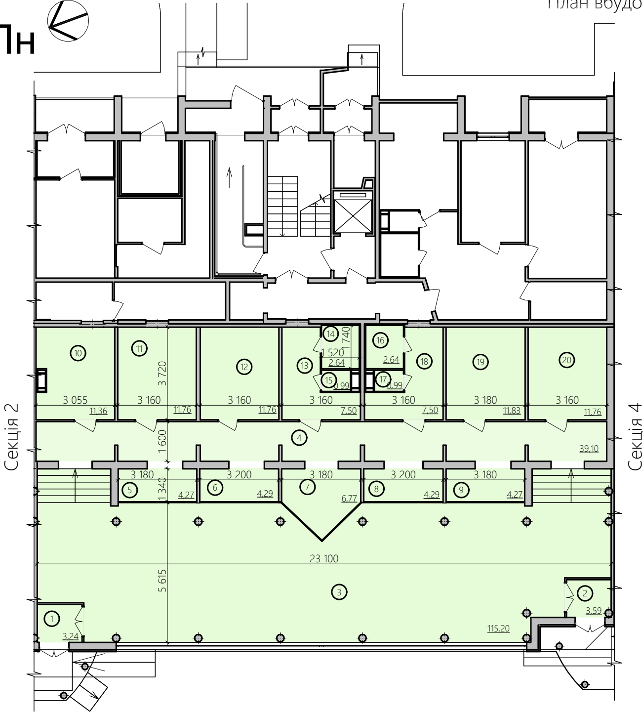
План вбудованих приміщень 3 секція
